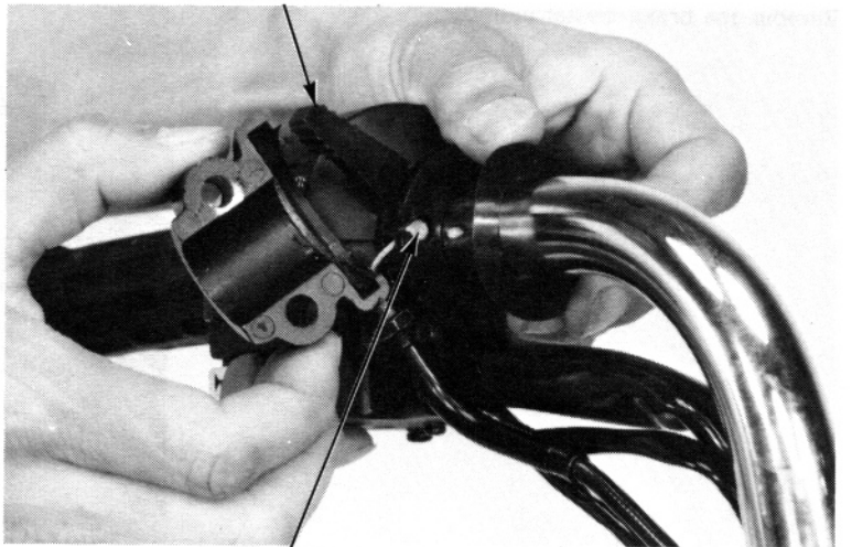
CHOKE CABLE
