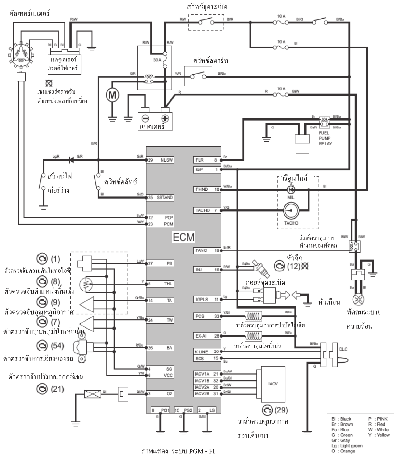
ภาพแสดง ระบบ PGM - FI
