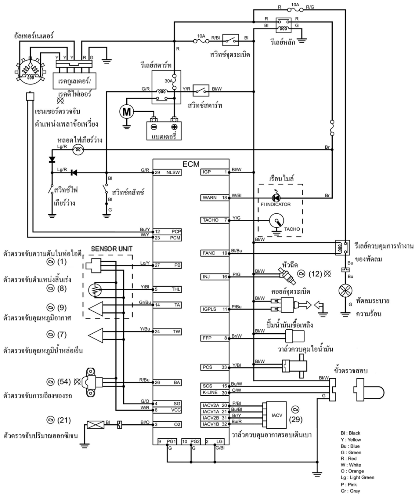
ภาพแสดง ระบบ PGM - FI
