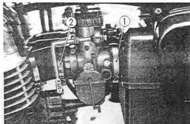
Fig. 6-3 ① Raccordement au filtre à air ② Collier isolant du carburateur
