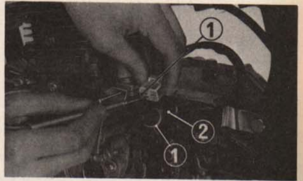
Fig. 4-90 (1) Conducteur vert clair/rouge (2) Contacteur de point mort
