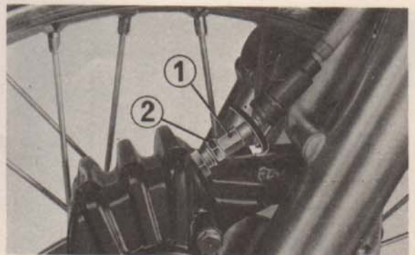
Fig. 4-29 (1) Boulon de réglage du câble (2) Contre-écrou
