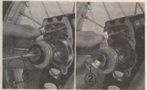
Fig. 4-27 (1) Tournevis ordinaire (2) Cliquet
