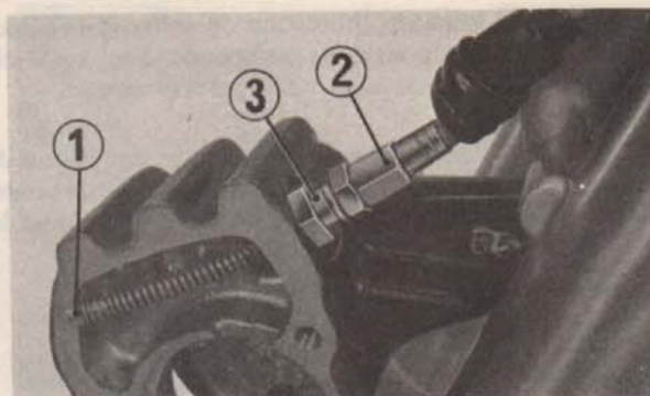
Fig. 4-22 (1) Extrémité de câble (2) Boulon de réglage (3) Boulon de réglage du câble
