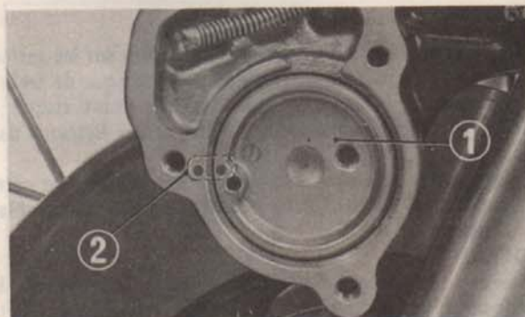
Fig. 4-25 (1) Plaquette d'étrier A (2) Repère de montage
