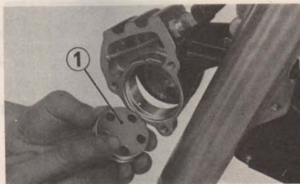
Fig. 4-24 (1) Mettre de la graisse au silicium KS62M au dos de la plaquette de frein B
