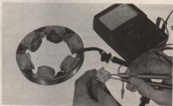
Fig. 3-87 Contrôle de l'état de la bobine fixe
