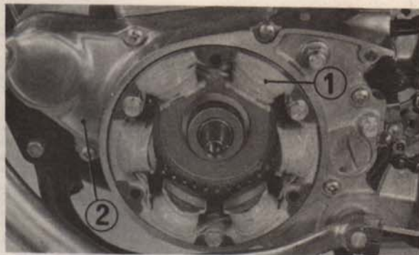
Fig. 3-86 (1) Carcasse d'alternateur (2) Couvercle de carter-moteur gauche
