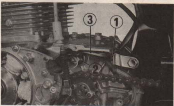
Fig. 3-88 (1) Rondelle isolante en caoutchouc (2) Contacteur de point mort (3) Conducteur d'alternateur
