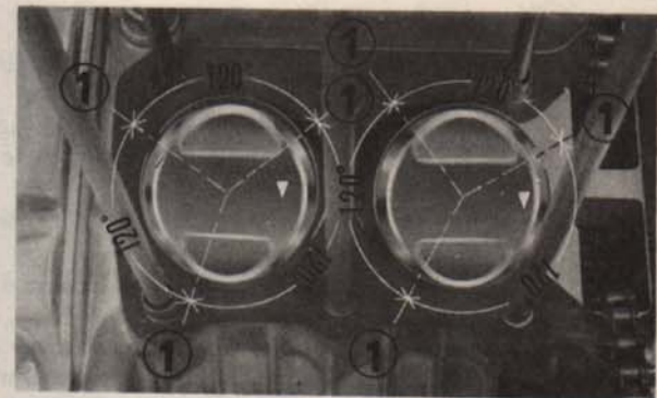
Fig. 3-27 (1) Espacement d'écartement de segments
