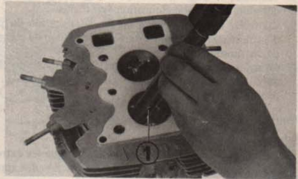
Fig. 3-12 (1) Extracteur de guide de soupape
