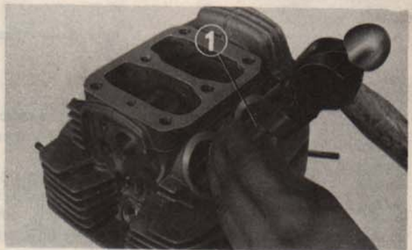
Fig. 3-13 (1) Outil de montage de guide de soupape
