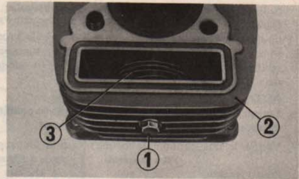
Fig. 3-11 (1) Boulon de fixation (2) Cylindre (3) Galet-guide de chaîne de distribution
