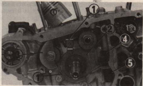
Fig. 3-10 (1) Plaquette d'arrêt (4) Tige de poussée (2) Tendeur (5) Ressort de tendeur (3) Galet de tendeur
