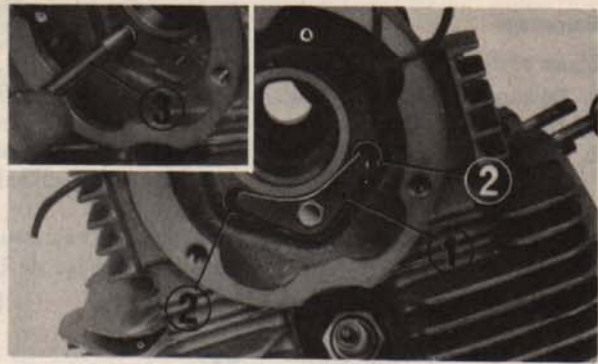
Fig. 3-7 (1) Arrêt d'axe de culbuteur (2) Axe de culbuteur (3) Boulon de 8mm
