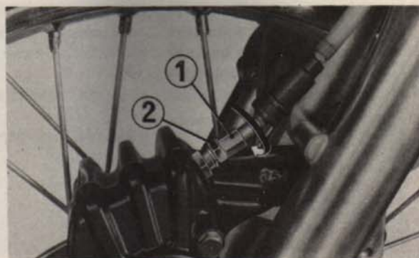
Fig. 2-18 (1) Boulon de réglage du câble de commande de frein (2) Contre-écrou
