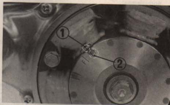
Fig. 2-1 (1) Index fixe (2) Repère "T"
