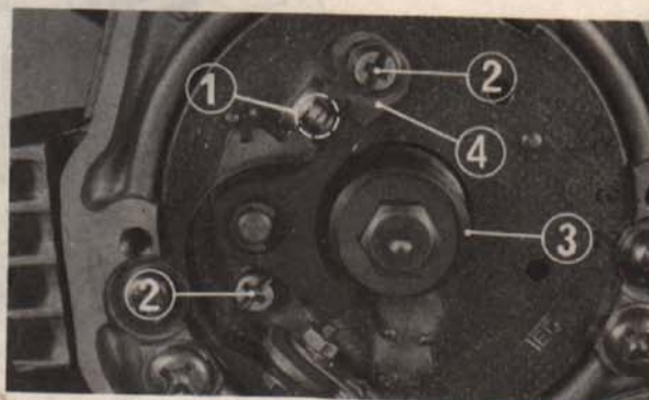
Fig. 2-3 (1) Vis platinees (2) Vis de blocage (3) Came de commande de vis platinees (4) Plateau des vis platinees
