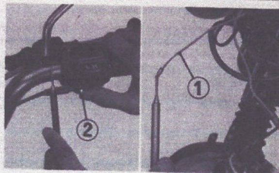
Fig. 4-89 (1) Jaune/rouge (2) Commutateur de démarreur
