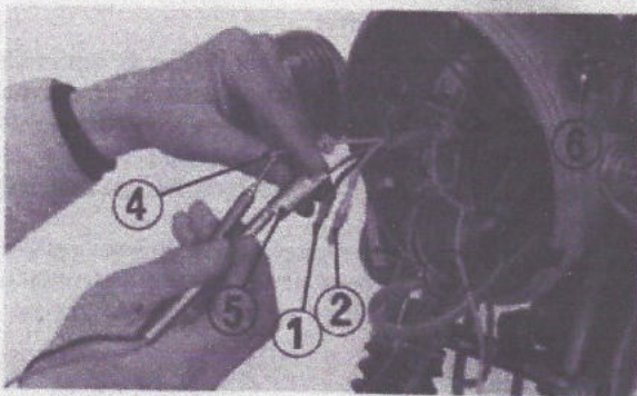
Fig. 4-87 (1) Noir (4) Jaune (2) Blanc/jaune (5) Brun/blanc (3) Brun/bleu (6) Interrupteur d'éclairage
