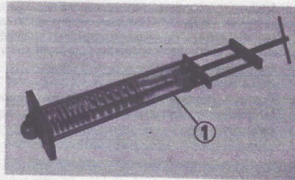
Fig. 4-67 (1) Outil de compression de ressort d'amortisseur arrière
