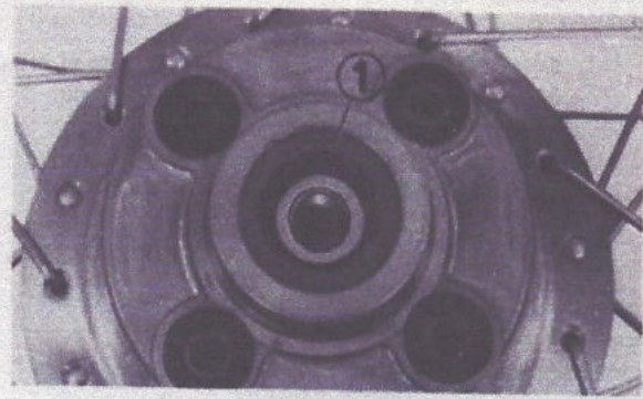
Fig. 4-57 (1) Joint d'étanchéité d'huile
