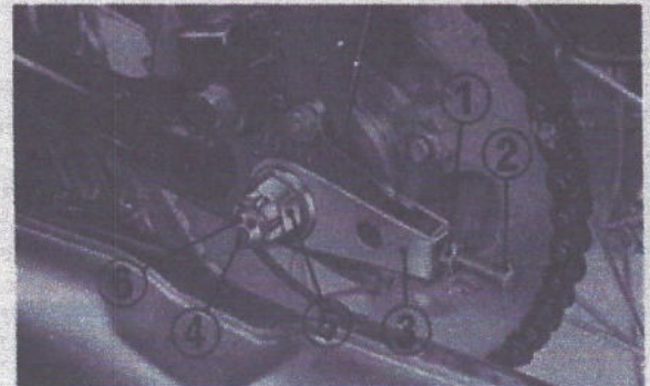
Fig. 4-55 (1) Contre-écrou (4) Goupille fendue (2) Boulon de réglage de chaîne de transmission (5) Ecrrou d'axe de roue arrière (3) Dispositif de réglage de chaîne de transmission (6) Axe de roue arrière
