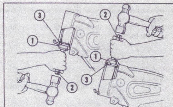
Fig. 4-41 (1) Accessoire de l'outil de montage de cuvette de retenue (2) Outil de montage de cuvette de retenue (3) Cuvette de retenue
