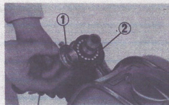
Fig. 4-42 (1) Cage de retenue à gorge supérieure (2) Billes d'acier
