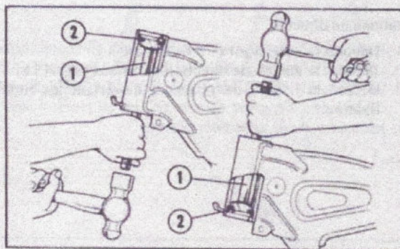
Fig. 4-40 (1) Extracteur de cage de retenue (2) Cage de retenue
