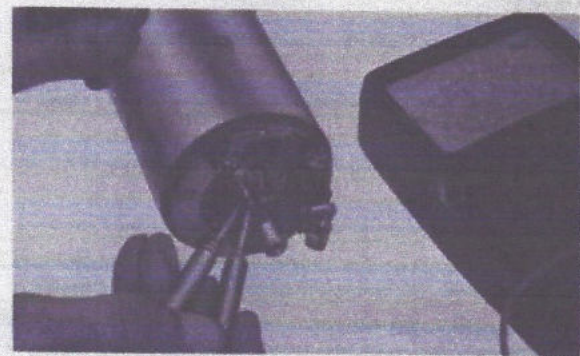
Fig. 3-107 Contrôle de l'état de l'enroulement d'induit
