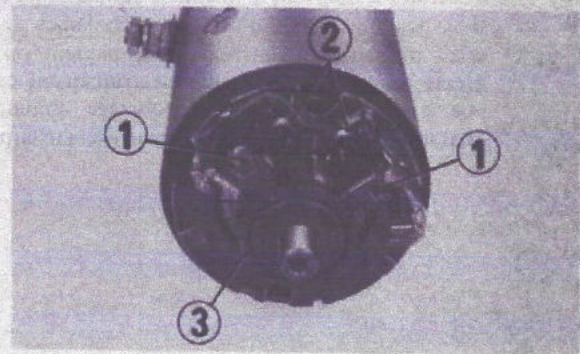
Fig. 3-105 (1) Balais (2) Ressort de balais (3) Collecteur
