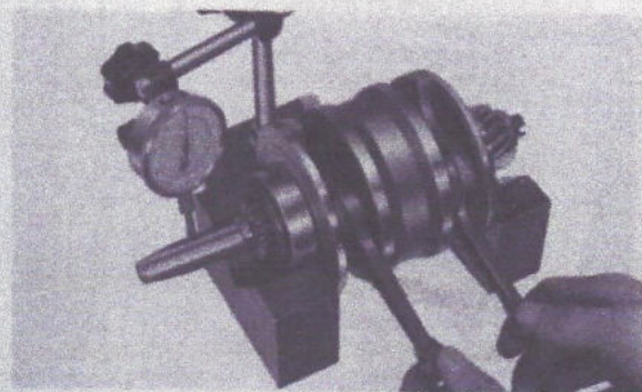
Fig. 3-33 Mesure d'usure de vilebrequin
