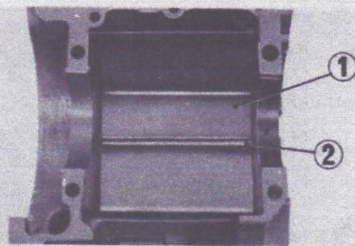
Fig. 3-32 (1) Séparateur d'huile (2) Tige d'assemblage
