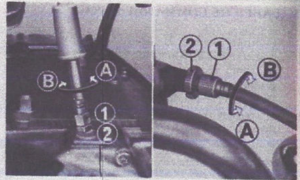
Fig. 2-12 (1) Molette de réglage (2) Contre-écrou
