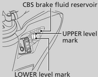
CBS brake
