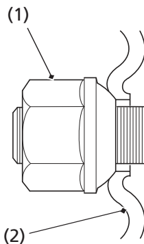
(2) wheel rim
