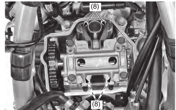
(8) rocker arms
