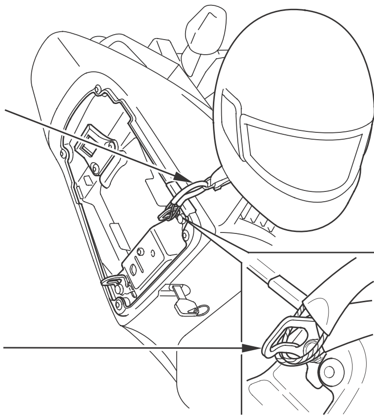
ヘルメットホルダ ヘルメットホルダワイヤ
