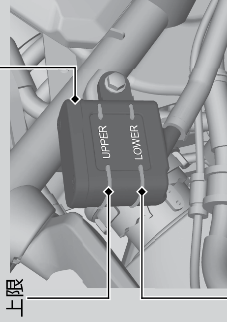
後輪ブレーキリザーバータンク
