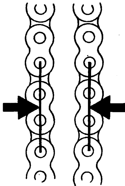
ドライブチェーンのたるみ
