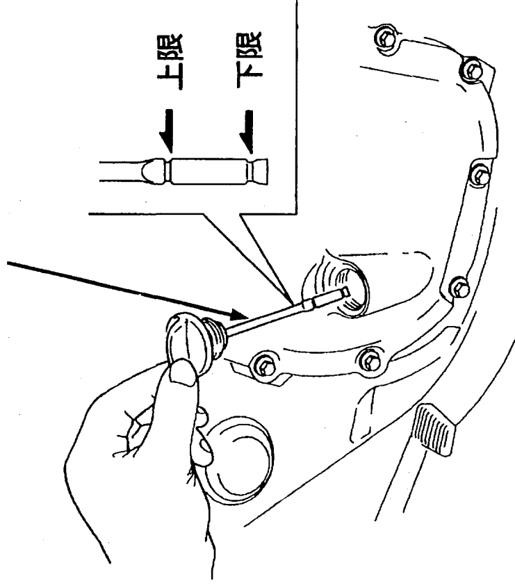
オイルレベルゲージ
