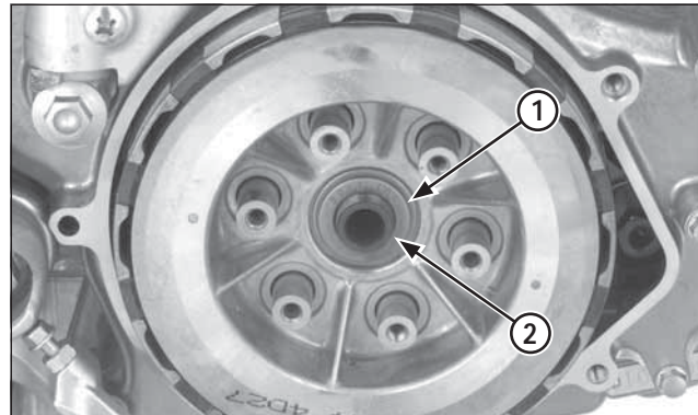
(1) RONDELLE-POUSSOIR (2) RONDELLE DE PRESSION (MARQUE "OUTSIDE" DEVANT)
