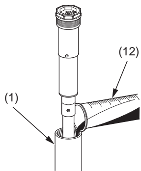
(1) gruppo della forcella (12) olio della forcella
