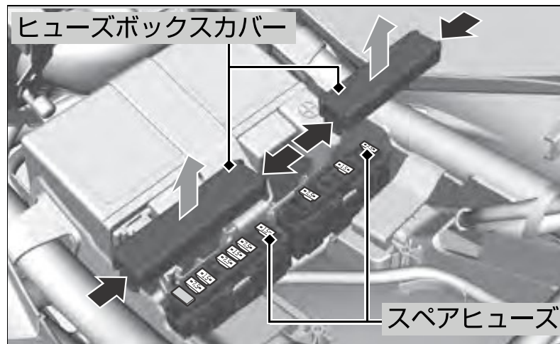
CBR400R<ABS>
