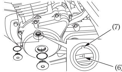
(6) T mark (7) Index mark
